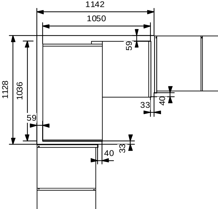
90° Ecke, 2-türig
