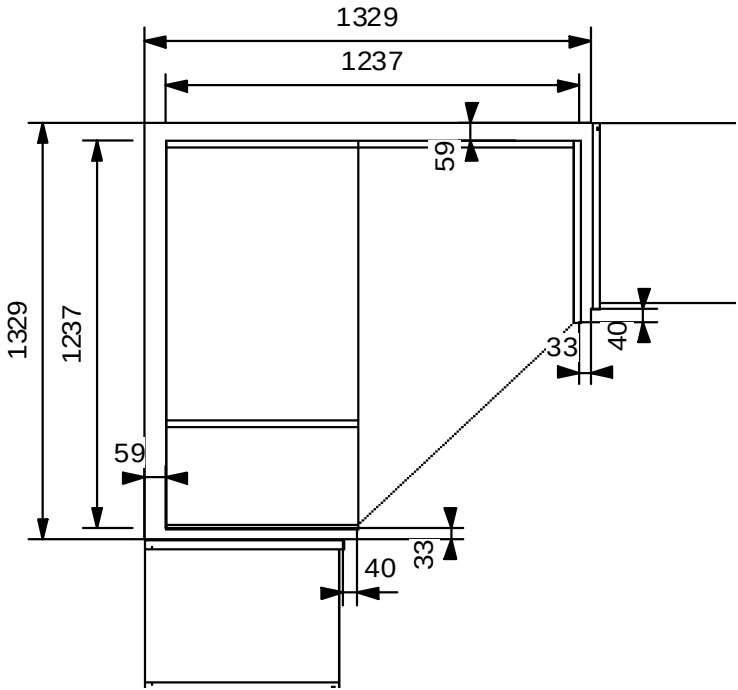
GRUNDSCHRANK
