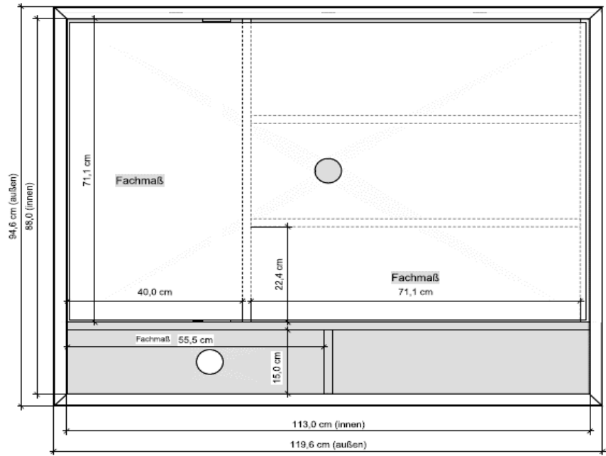
Paneel schwenkbar links oder rechts
